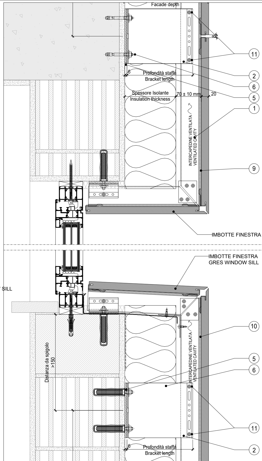
V2 SEZIONE VERTICALE CIELINO E BANCALE IN GRESS - VERTICAL SECTION SISTEMA INVISIBILE WALLTECH- INVISIBLE SYSTEM WALLTECH
