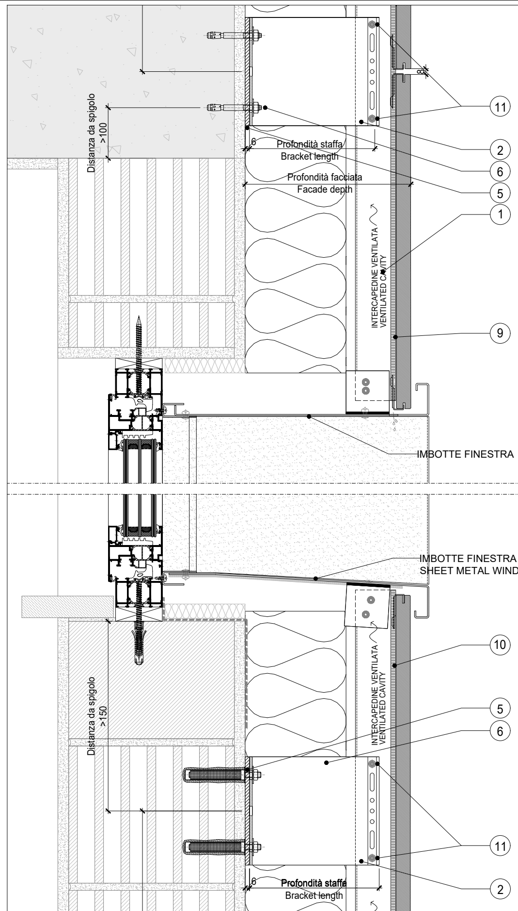
V1 SEZIONE VERTICALE CIELINO E BANCALE IN LAMIERA - VERTICAL SECTION SISTEMA INVISIBILE WALLTECH- INVISIBLE SYSTEM WALLTECH
