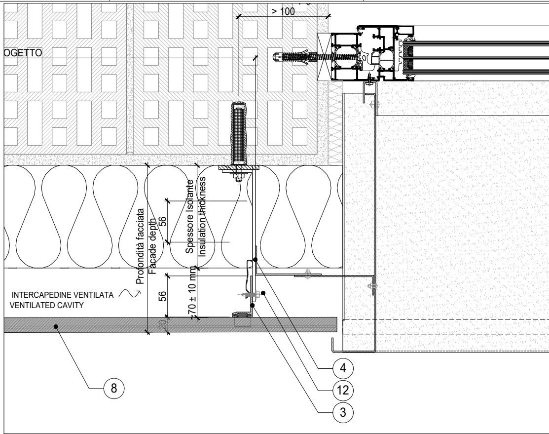
H2 SEZIONE ORIZZONTALE SPALLA LAMIERA -HORIZONTAL SECTION SISTEMA INVISIBILE WALLTECH- INVISIBLE SYSTEM WALLTECH
