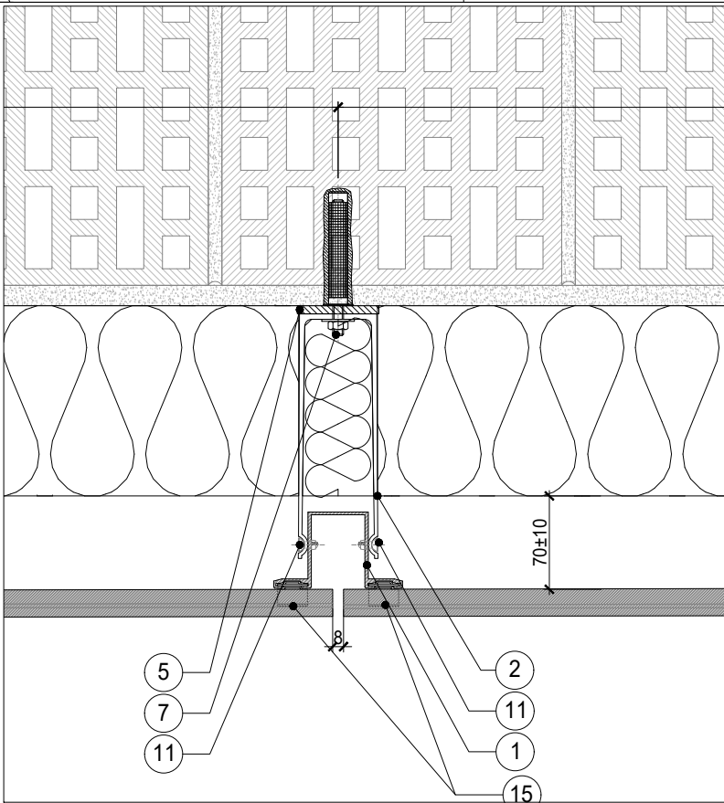
H1 SEZIONE ORIZZONTALE TIPICA- HORIZONTAL SECTION SISTEMA INVISIBILE WALLTECH- INVISIBLE SYSTEM WALLTECH
