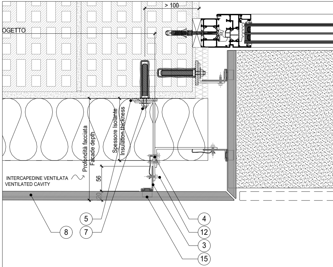
H3 SEZIONE ORIZZONTALE SPALLA GRESS-HORIZONTAL SECTION SISTEMA INVISIBILE WALLTECH- INVISIBLE SYSTEM WALLTECH
