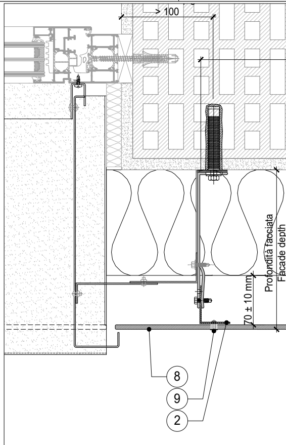
H3 SEZIONE ORIZZONTALE SPALLA GRESS - HORIZONTAL SECTION SISTEMA VISTA GresX - VISIBLE SYSTEM GresX
