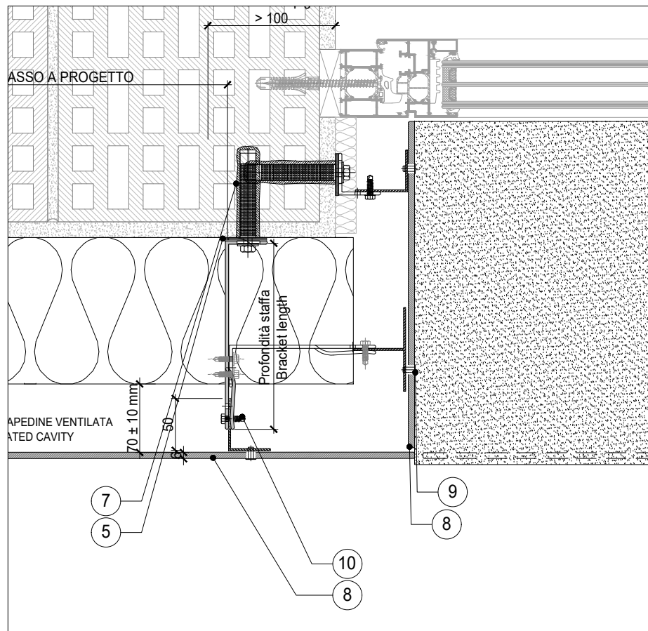
H5 SEZIONE ORIZZONTALE SPALLA GRESS - HORIZONTAL SECTION SISTEMA VISTA GresX - VISIBLE SYSTEM GresX
