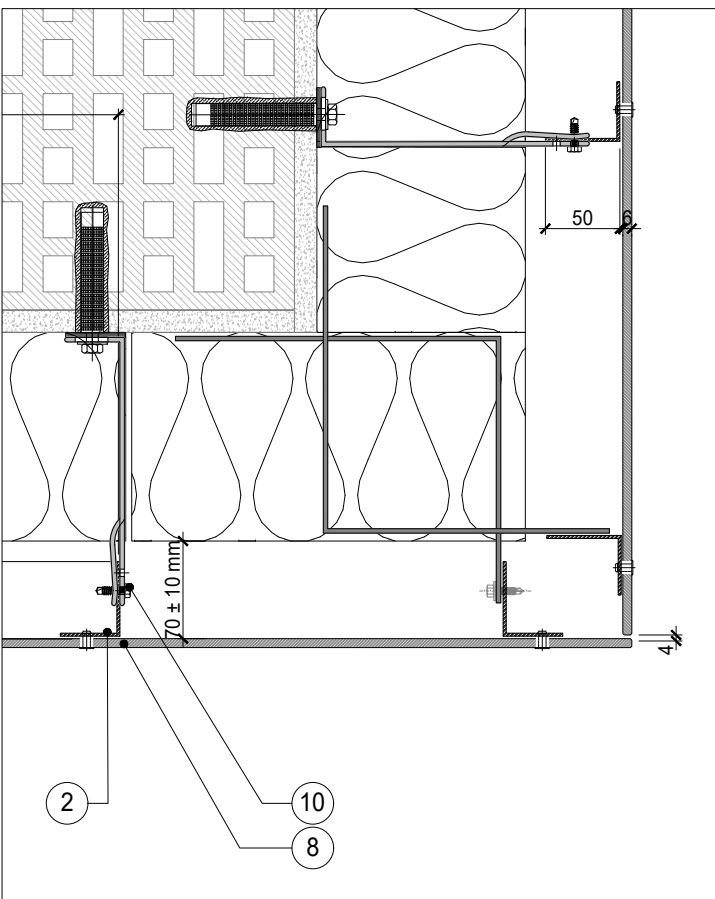
H7 SEZIONE ORIZZONTALE SPALLA GRESS - HORIZONTAL SECTION SISTEMA VISTA GresX - VISIBLE SYSTEM GresX
