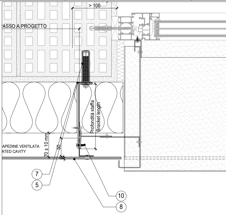
H2 SEZIONE ORIZZONTALE SPALLA LAMIERA - HORIZONTAL SECTION SISTEMA VISTA GresX - VISIBLE SYSTEM GresX
