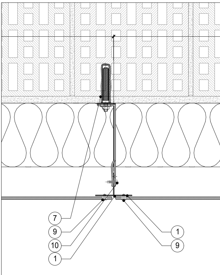
H4 SEZIONE ORIZZONTALE ANGOLO - HORIZONTAL SECTION SISTEMA VISTA GresX - VISIBLE SYSTEM GresX
