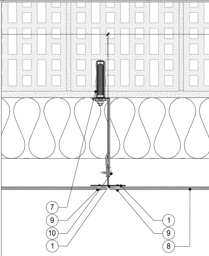
H1 SEZIONE ORIZZONTALE TIPICA - HORIZONTAL SECTION SISTEMA VISTA GresX - VISIBLE SYSTEM GresX
