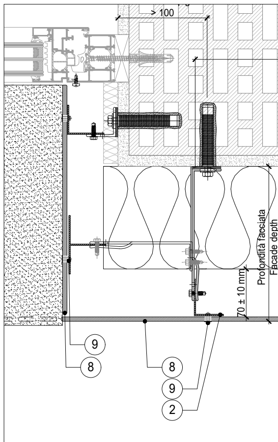
H6 SEZIONE ORIZZONTALE SPALLA GRESS - HORIZONTAL SECTION SISTEMA VISTA GresX - VISIBLE SYSTEM GresX
