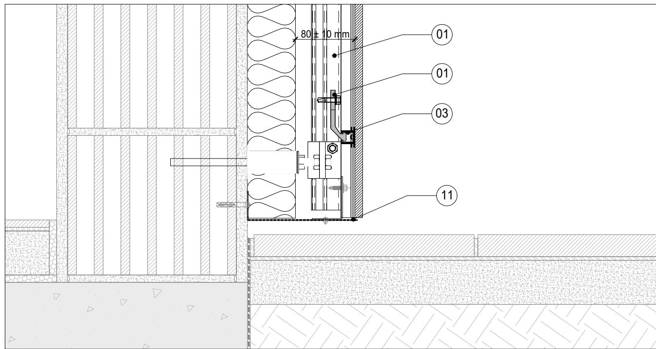
V2 SEZIONE VERTICALE TIPICA - VERTICLA SECTION SISTEMA INVISIBLE FLEX 5 - INVISIBLE SYSTEM FLEX 5
