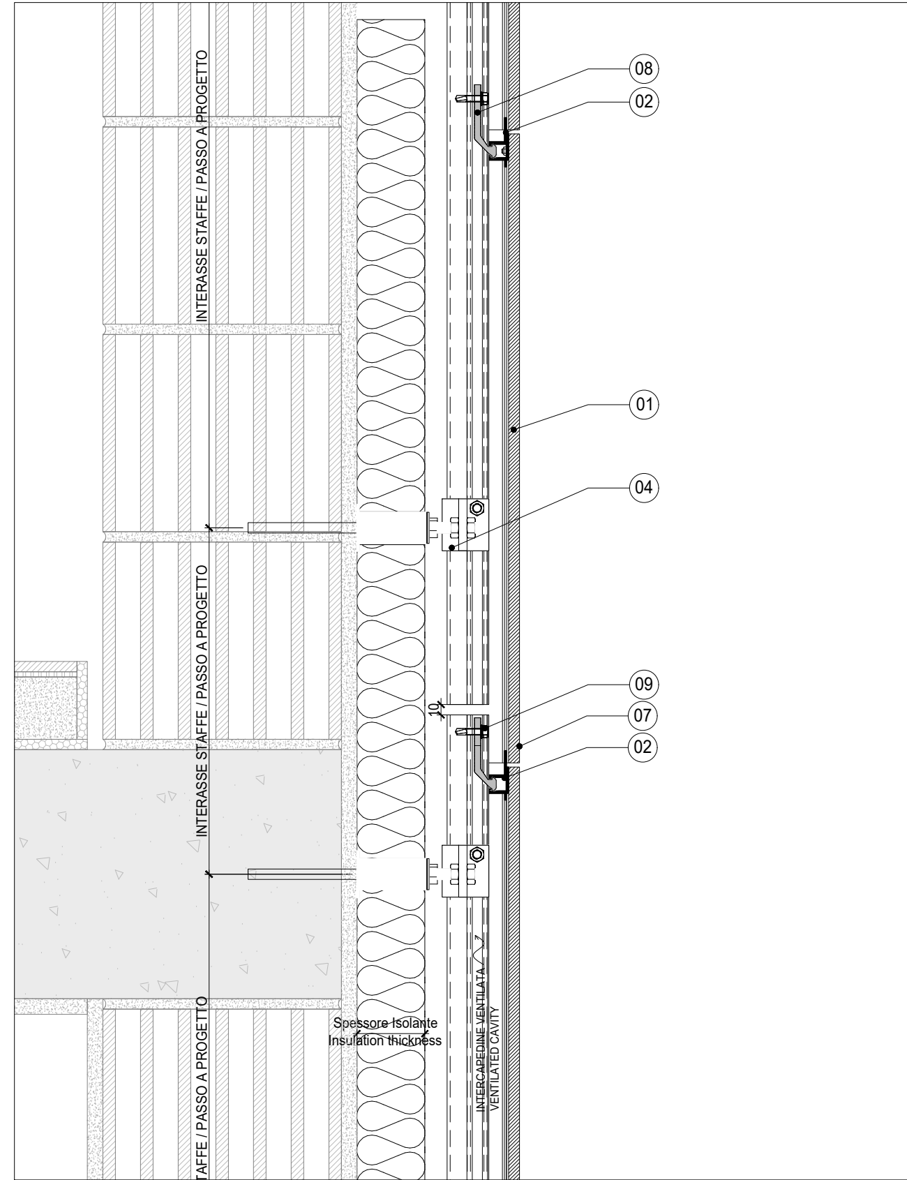
V2 SEZIONE VERTICALE TIPICA - VERTICLA SECTION SISTEMA INVISIBLE FLEX 5 - INVISIBLE SYSTEM FLEX 5
