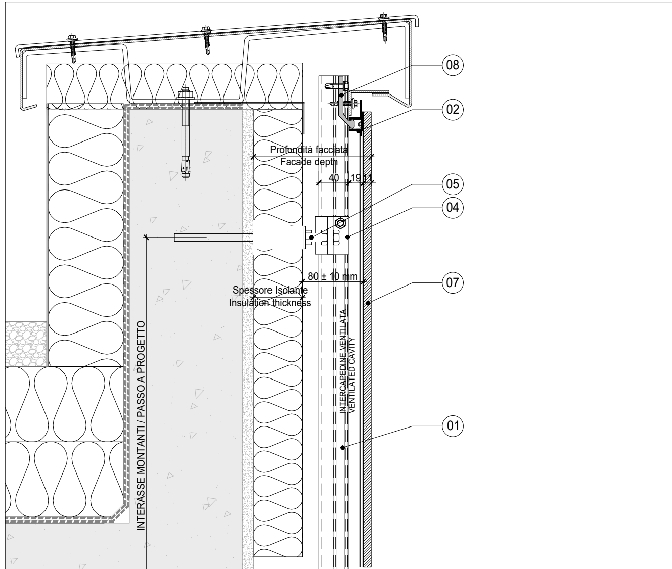
V1 SEZIONE VERTICALE SU LATTONERIA DI SOMMITA'- VERTICLA SECTION SISTEMA INVISIBLE FLEX 5 - INVISIBLE SYSTEM FLEX 5
