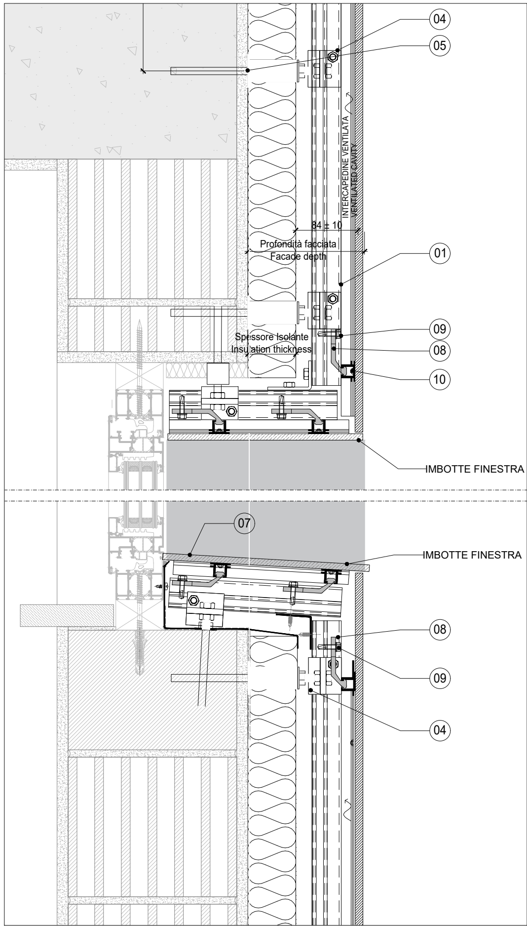
V2 SEZIONE VERTICALE CIELINO E BANCALE IN GRESS - VERTICAL SECTION SISTEMA INVISIBLE FLEX 5 - INVISIBLE SYSTEM FLEX 5
