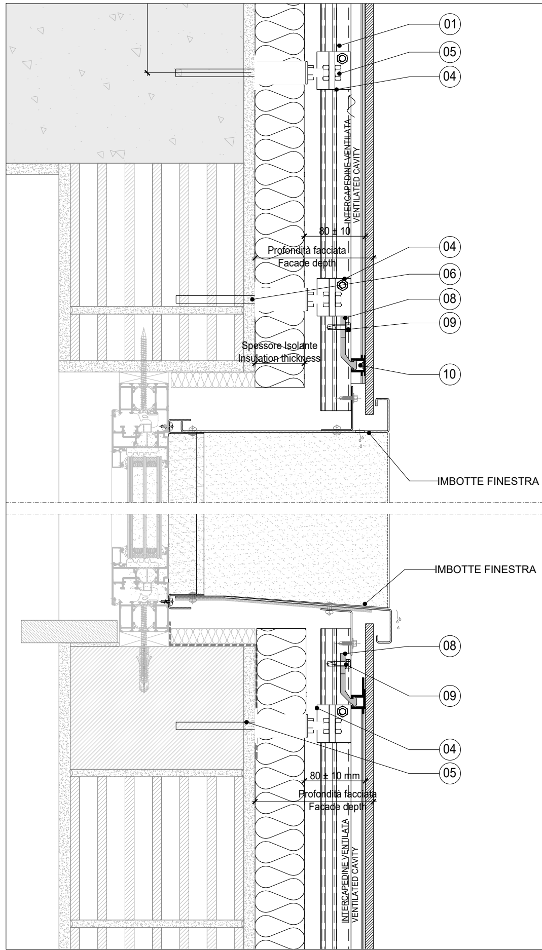
V1 SEZIONE VERTICALE CIELINO E BANCALE IN LAMIERA - VERTICAL SECTION SISTEMA INVISIBLE FLEX 5 - INVISIBLE SYSTEM FLEX 5
