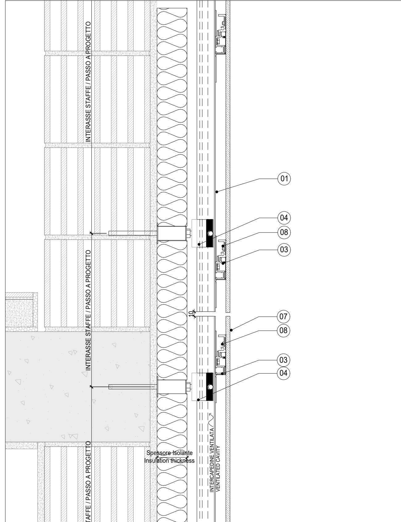
V3 SEZIONE VERTICALE PARTENZA FACCIATA- VERTICAL SECTION SISTEMA INVISIBLE FLEX 3 - INVISIBLE SYSTEM FLEX 3
