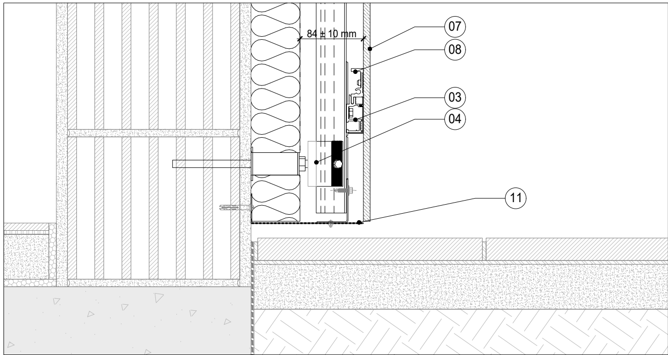
V2 SEZIONE VERTICALE TIPICA - VERTICAL SECTION SISTEMA INVISIBLE FLEX 3 - INVISIBLE SYSTEM FLEX 3
