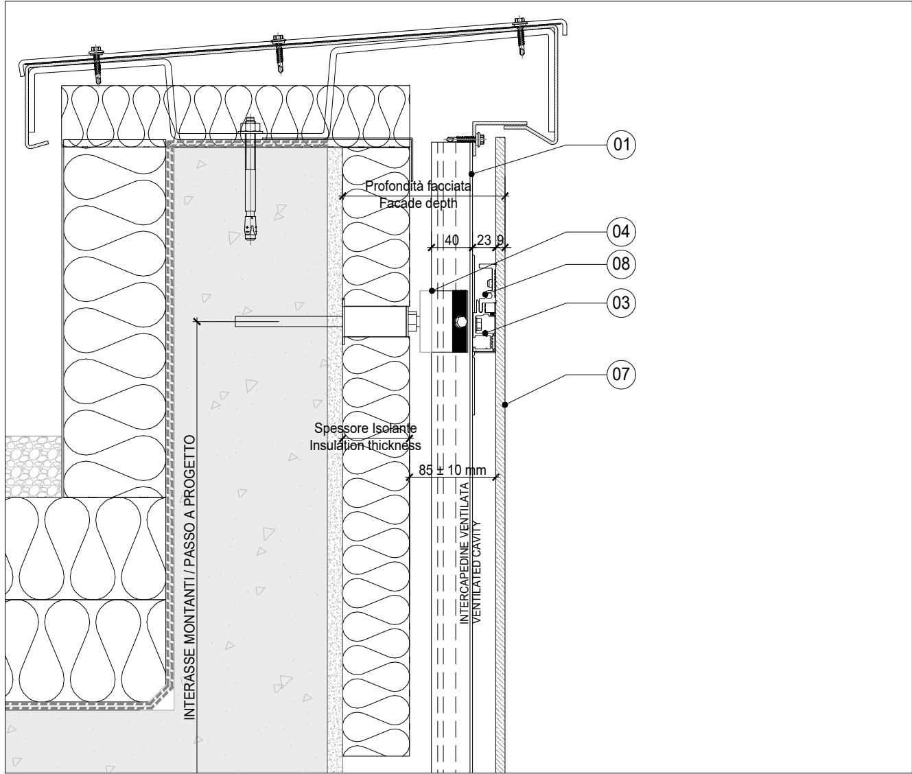
V1 SEZIONE VERTICALE SU LATTONERIA DI SOMMITA'- VERTICAL SECTION SISTEMA INVISIBLE FLEX 3 - INVISIBLE SYSTEM FLEX 3
