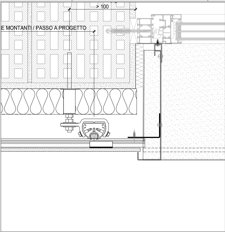
H2 SEZIONE ORIZZONTALE SPALLA LAMIERA - HORIZONTAL SECTION SISTEMA INVISIBILE FLEX 3 - INVISIBLE SYSTEM FLEX 3
