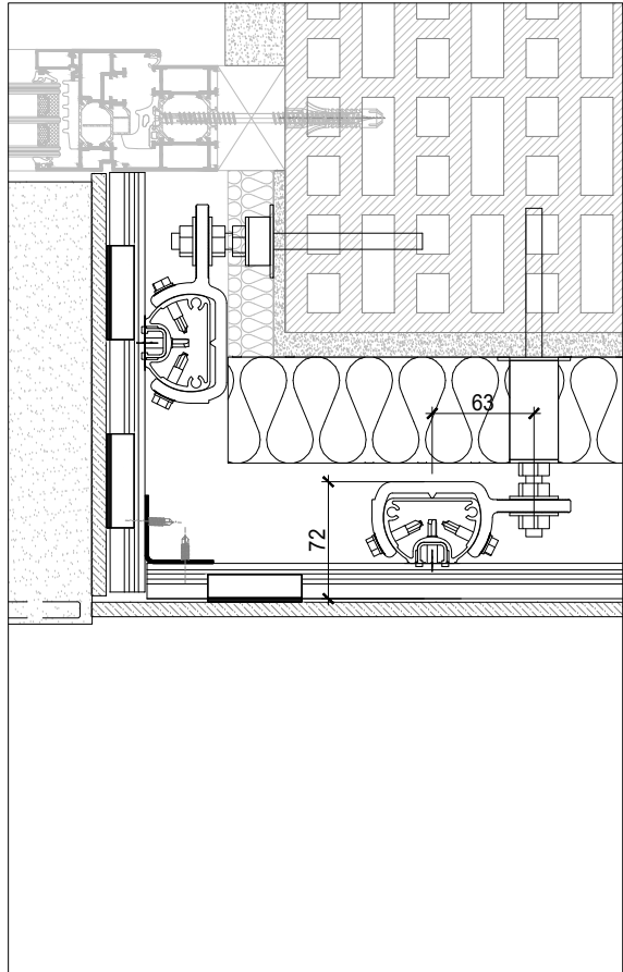
H6 SEZIONE ORIZZONTALE ANGOLO - HORIZONTAL SECTION SISTEMA INVISIBILE FLEX 3 - INVISIBLE SYSTEM FLEX 3
