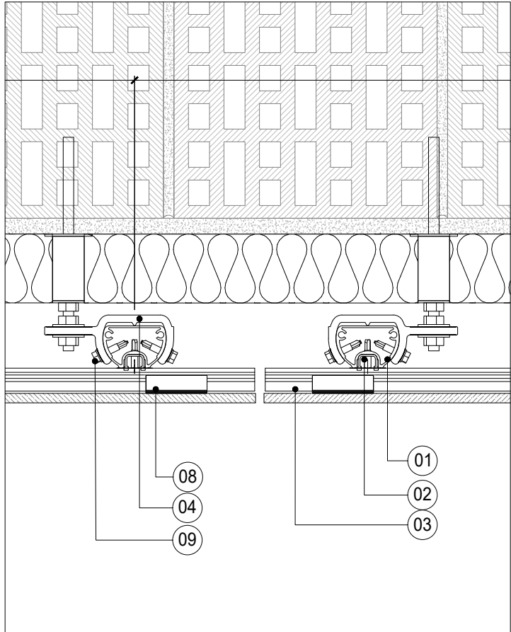
H4 SEZIONE ORIZZONTALE ANGOLO - HORIZONTAL SECTION SISTEMA INVISIBILE FLEX 3 - INVISIBLE SYSTEM FLEX 3
