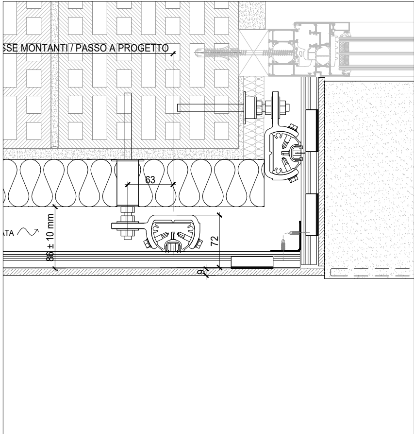
H5 SEZIONE ORIZZONTALE ANGOLO - HORIZONTAL SECTION SISTEMA INVISIBILE FLEX 3 - INVISIBLE SYSTEM FLEX 3
