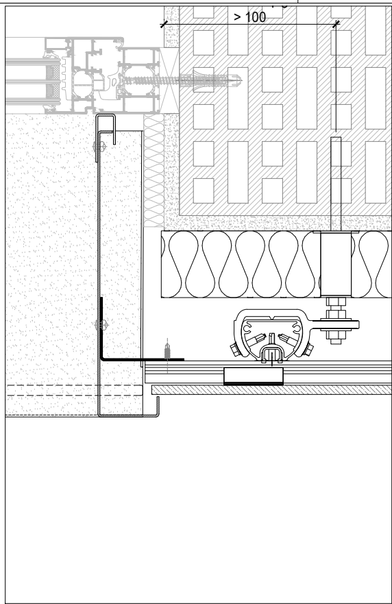
H3 SEZIONE ORIZZONTALE SPALLA LAMIERA - HORIZONTAL SECTION SISTEMA INVISIBILE FLEX 3 - INVISIBLE SYSTEM FLEX 3
