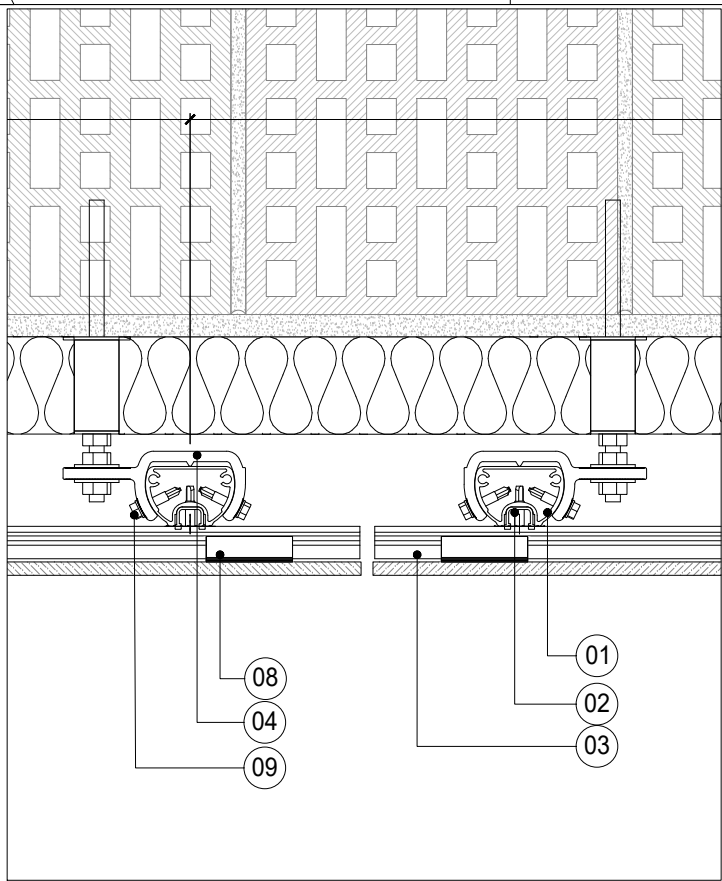
H1 SEZIONE ORIZZONTALE TIPICA - HORIZONTAL SECTION SISTEMA INVISIBILE FLEX 3 - INVISIBLE SYSTEM FLEX 3
